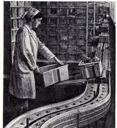
Рис. 2. Конвейер для транспортирования ящиков с письмами с автоматической выгрузкой их согласно адресу (СССР).
